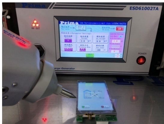
图 4-2 ESD 测试图
