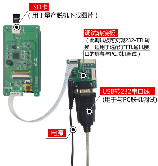
图 1-5 调试工具图
