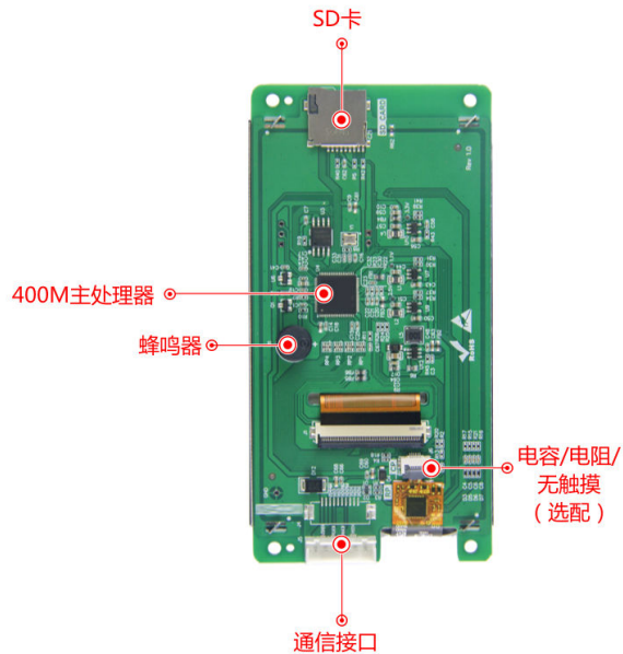
图 1-4 硬件配置图
