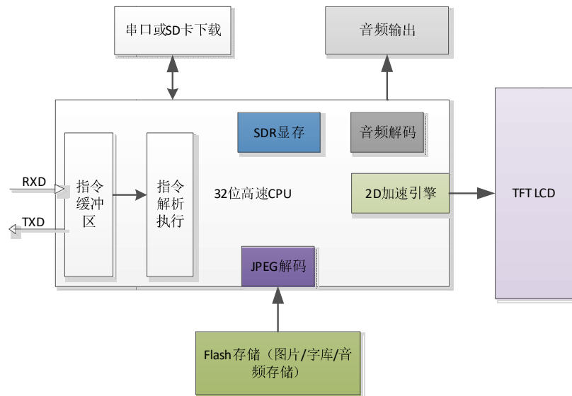
图 8-1 M 系列串口屏内部结构图
