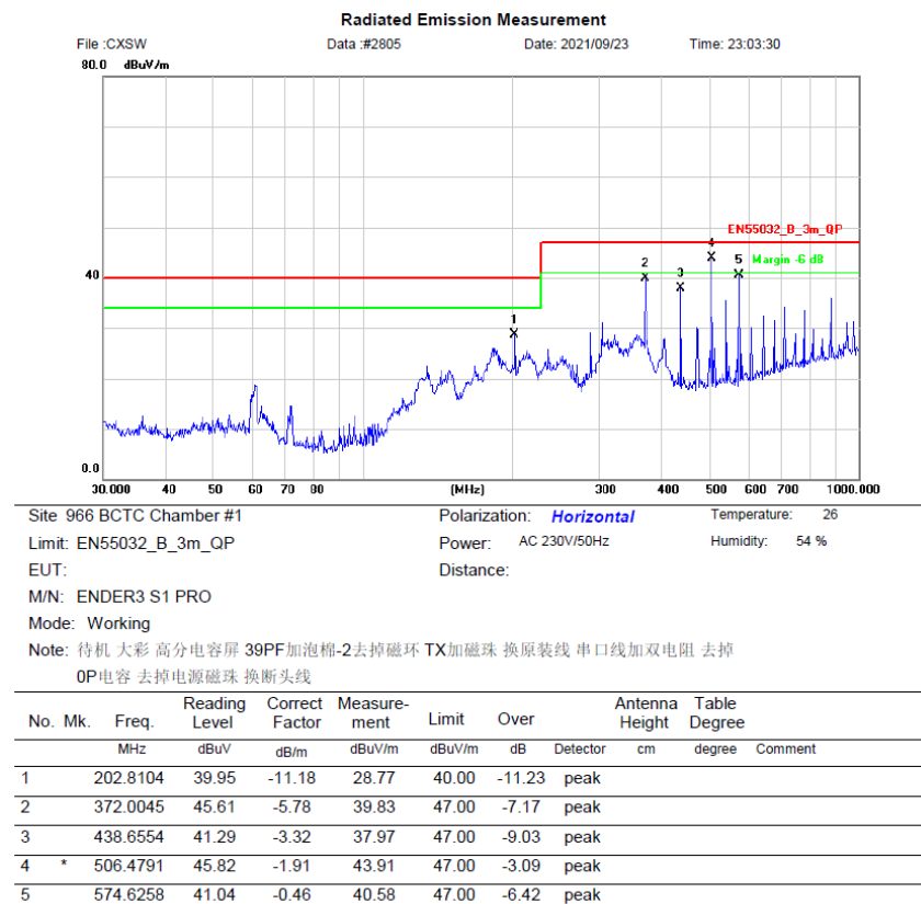
图 4-5 辐射测试水平方向
