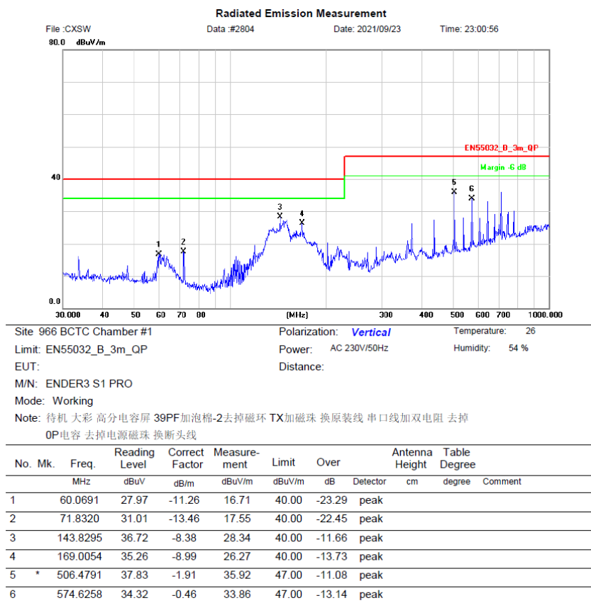
图 4-6 辐射测试垂直方向
