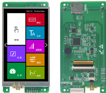
图 1-2 4.3 寸电阻触摸参考图
