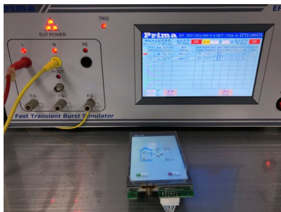
图 4-3 群脉冲测试图
