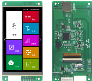
图 1-3 4.3 寸无触摸参考图
